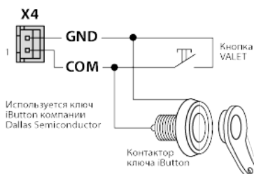
Подключение контактора ключа iButton
